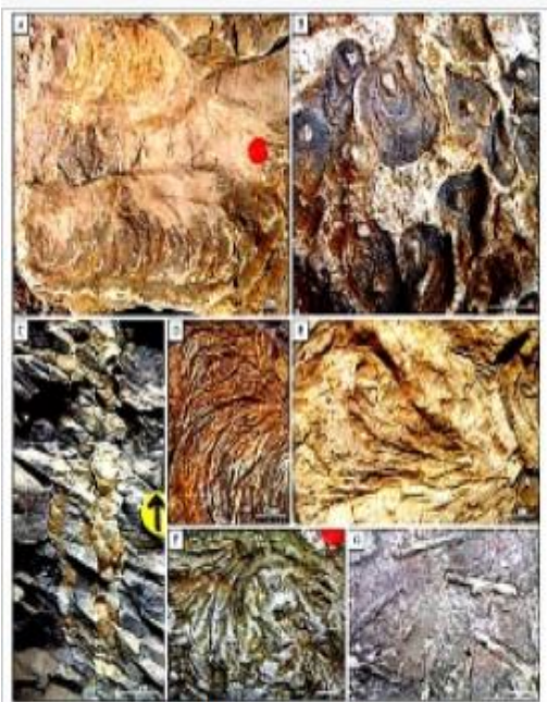
贵州独山泥盆系剖面遗迹化石
