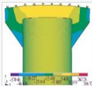
预应力加固后主应力云图
